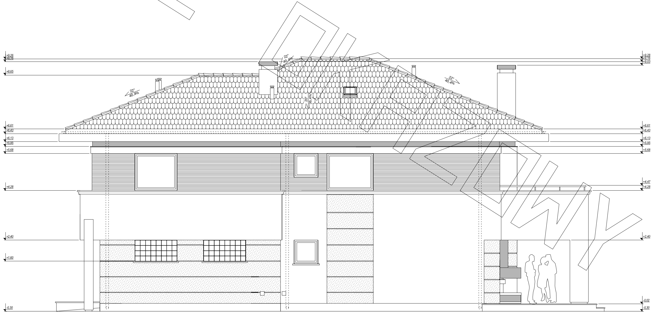
elewacja boczna
