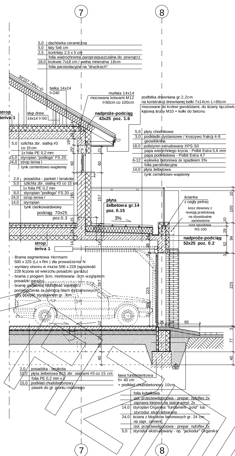
Przekrój B'-B'
