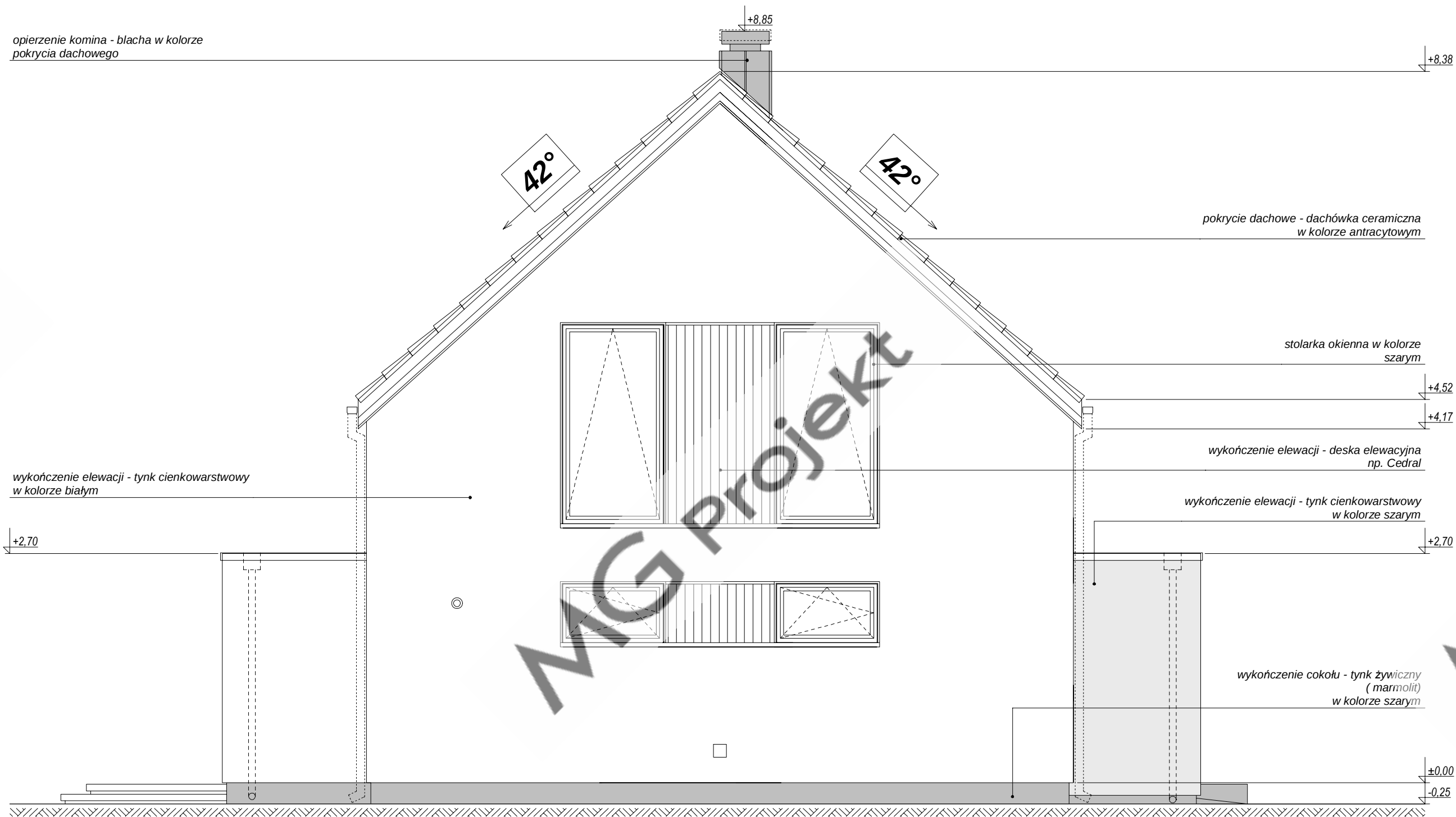
ELEWACJA BOCZNA
