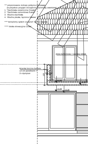
WIDOK ŚCIANY ELEWACJI TYLNEJ ( balkon , oraz podciąg podcienia )
