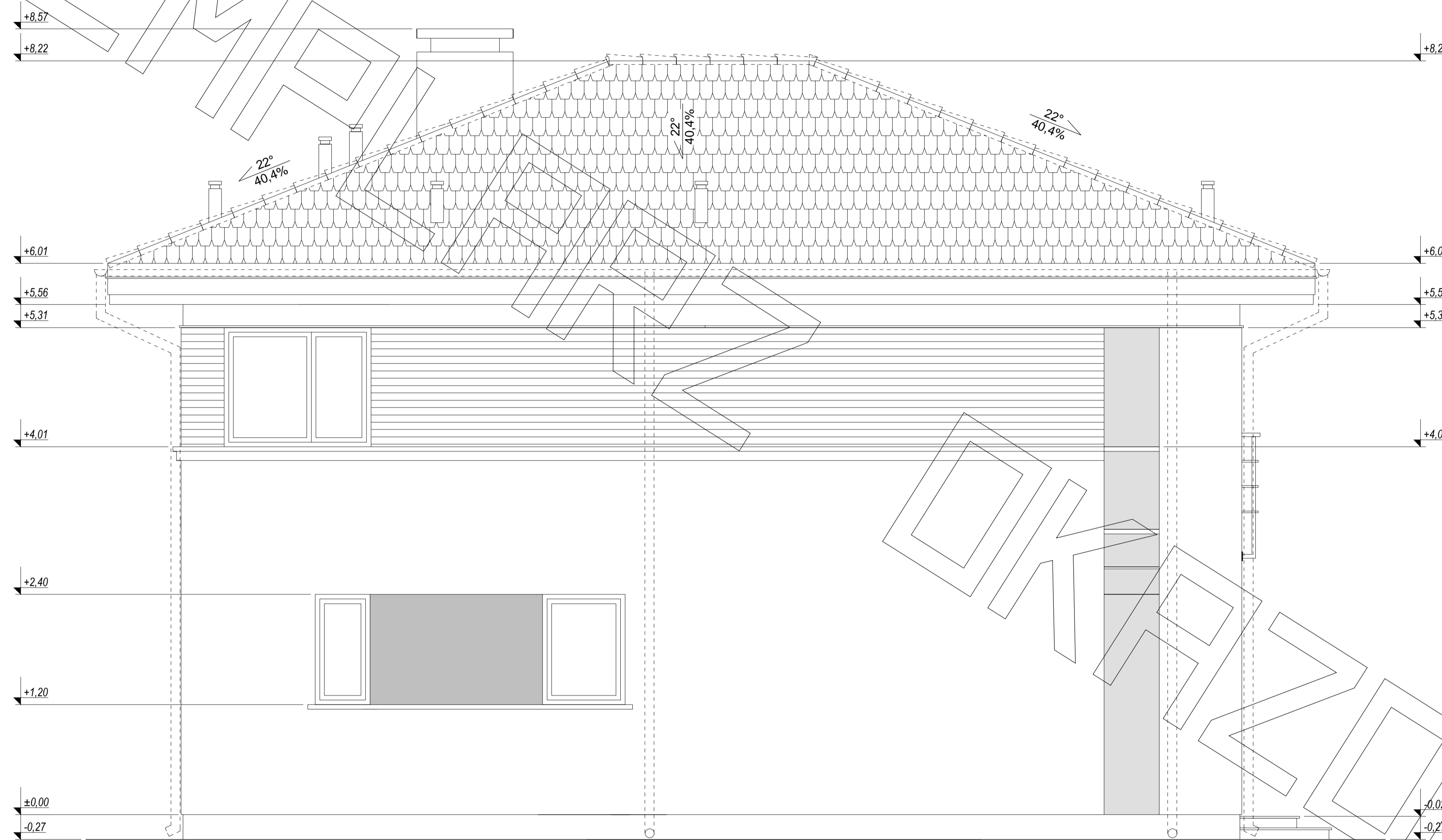
elewacja tylna :
