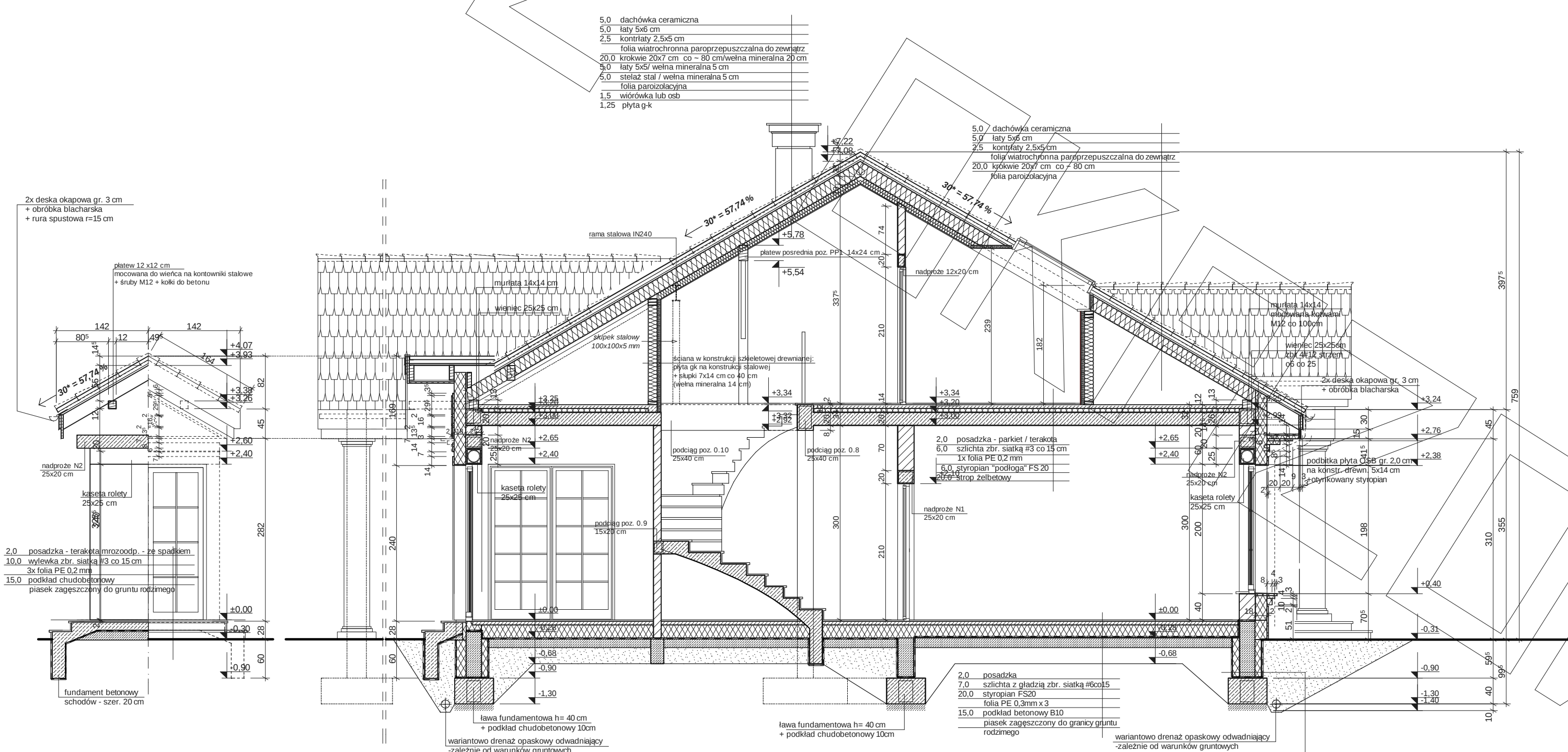
PRZEKRÓJ B-B
