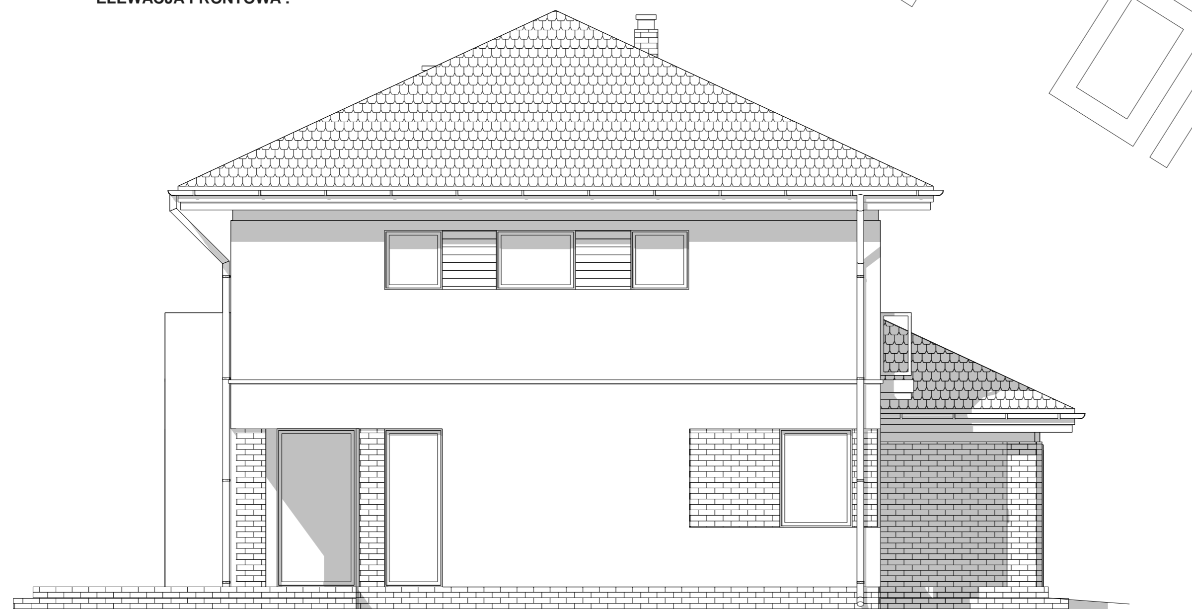
ELEWACJA BOCZNA :
