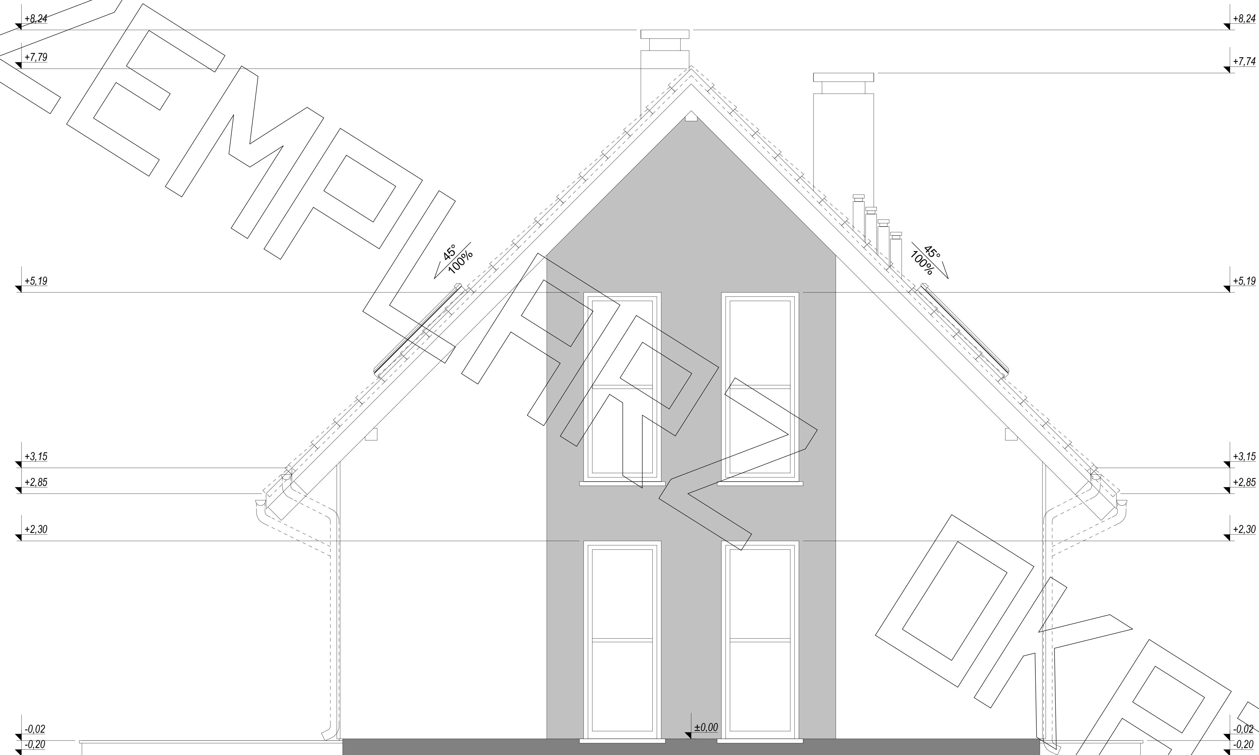
elewacja boczna :
