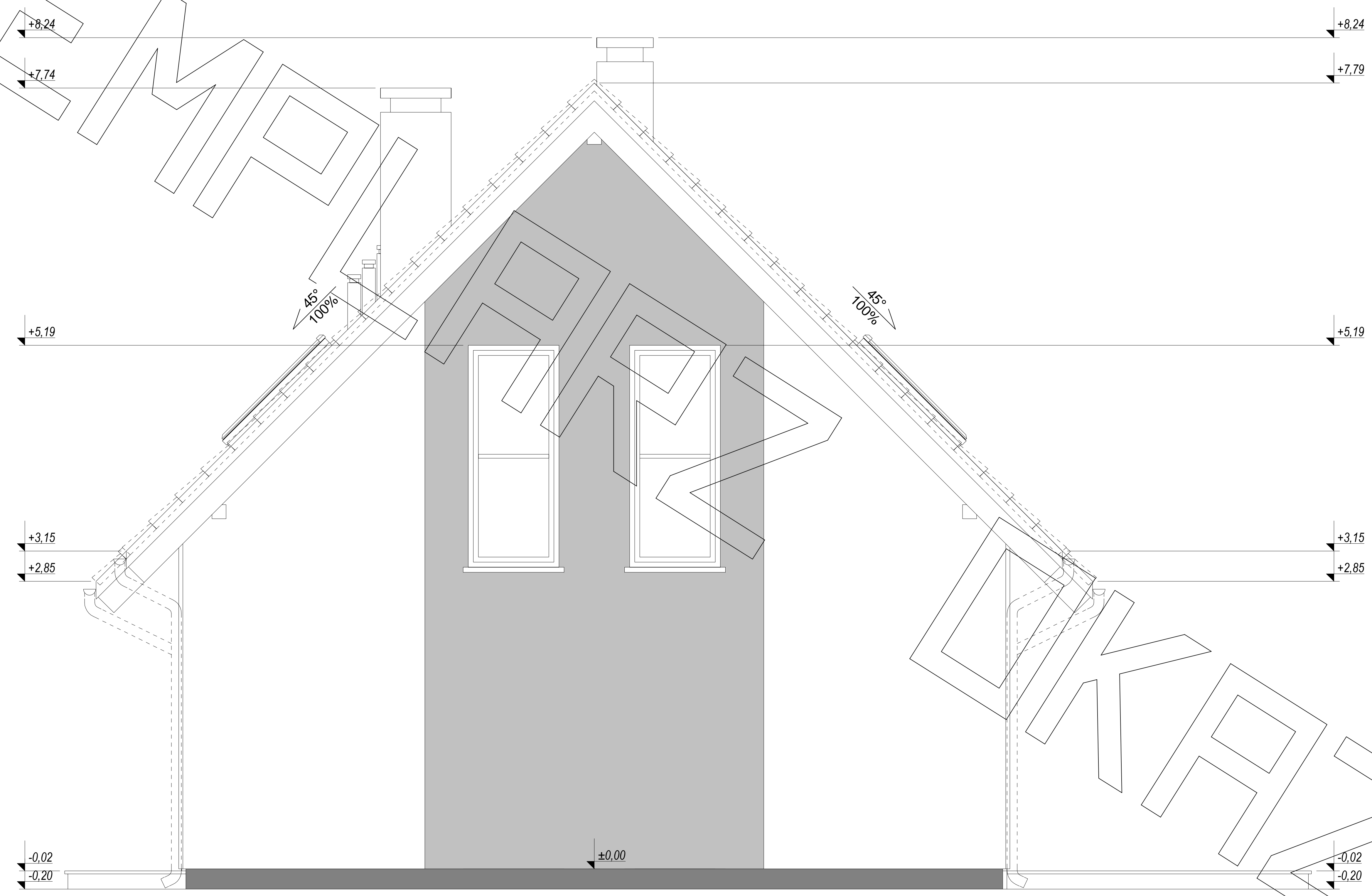
elewacja boczna :
