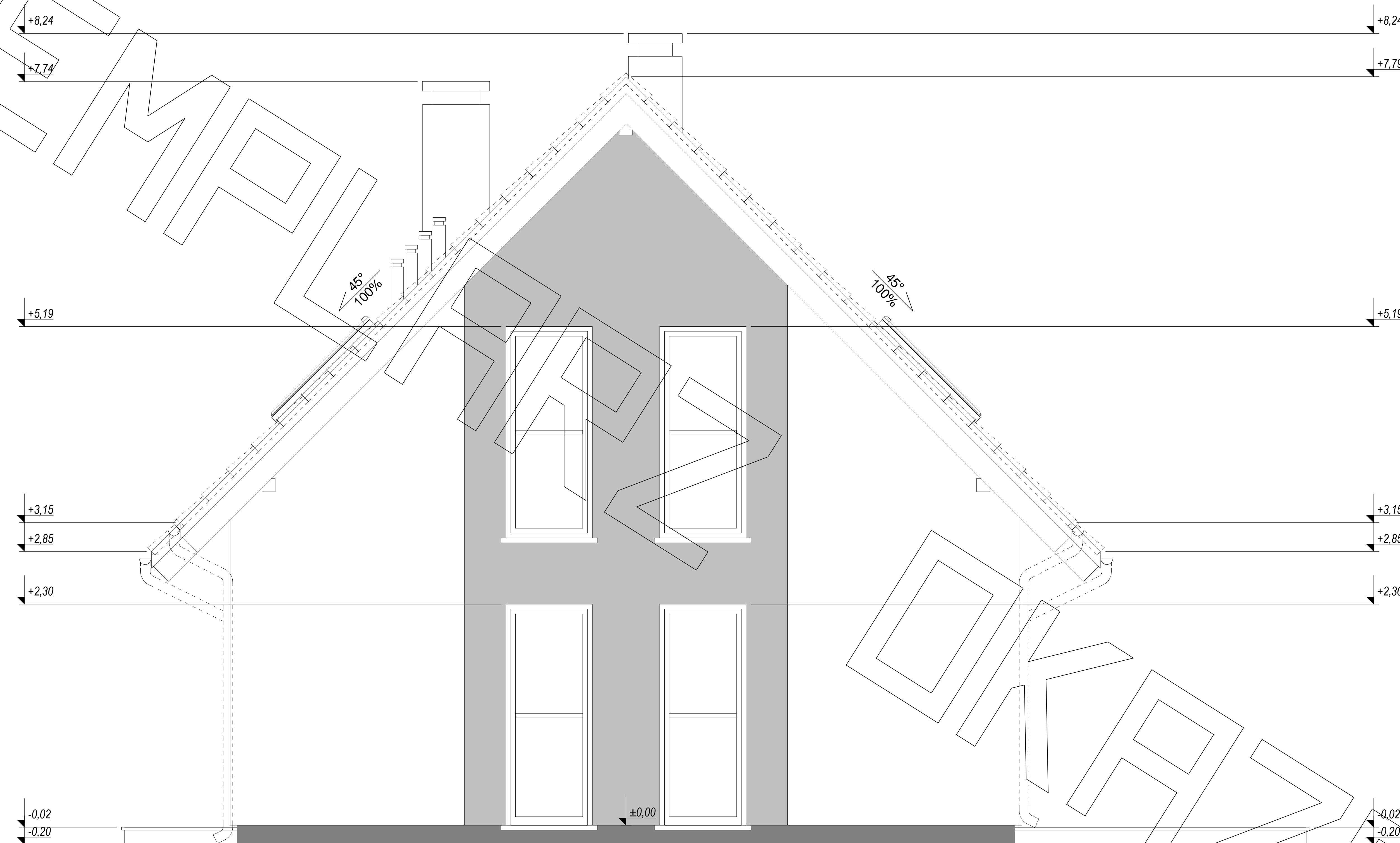
elewacja boczna :
