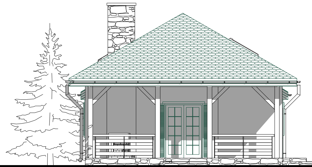
ELEWACJA OGRODOWA
