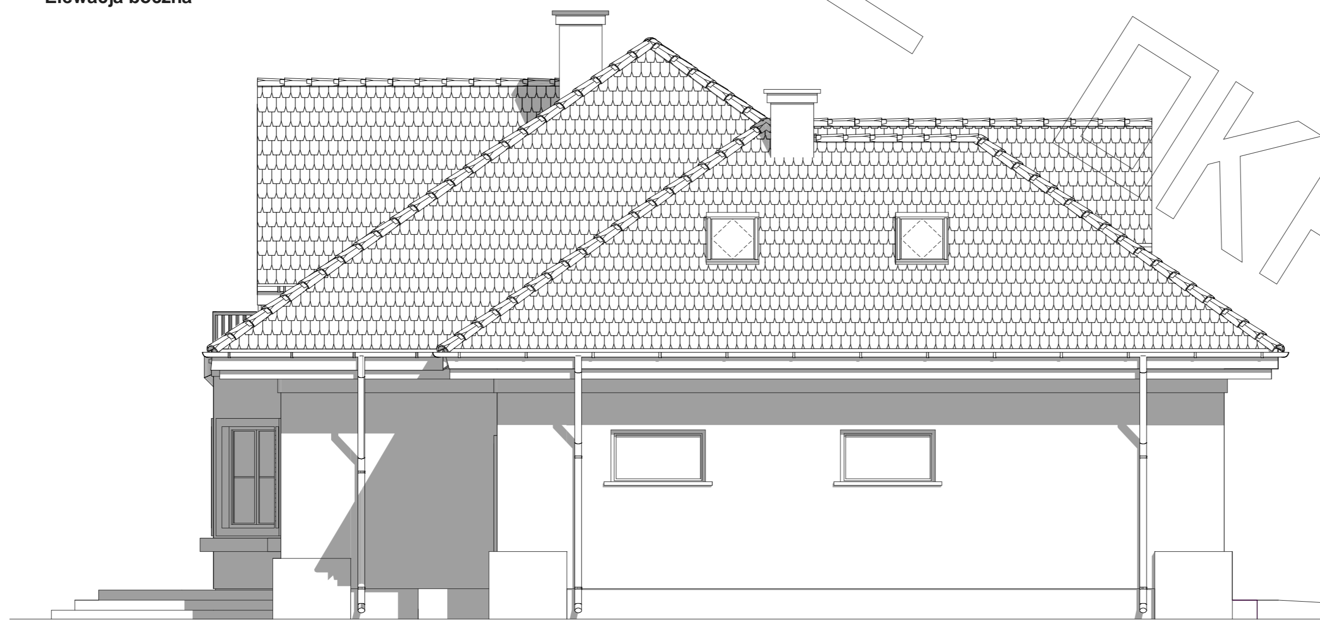
Elewacja boczna
