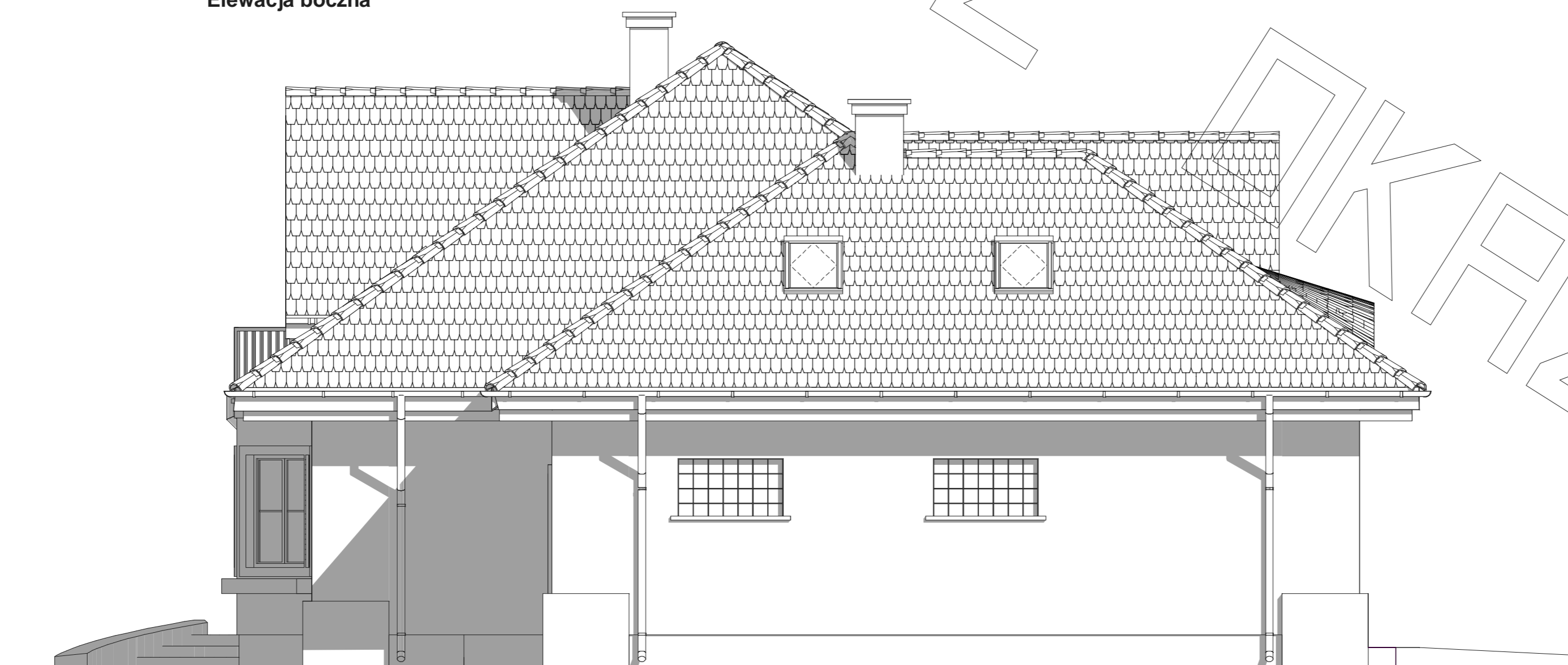
Elewacja boczna
