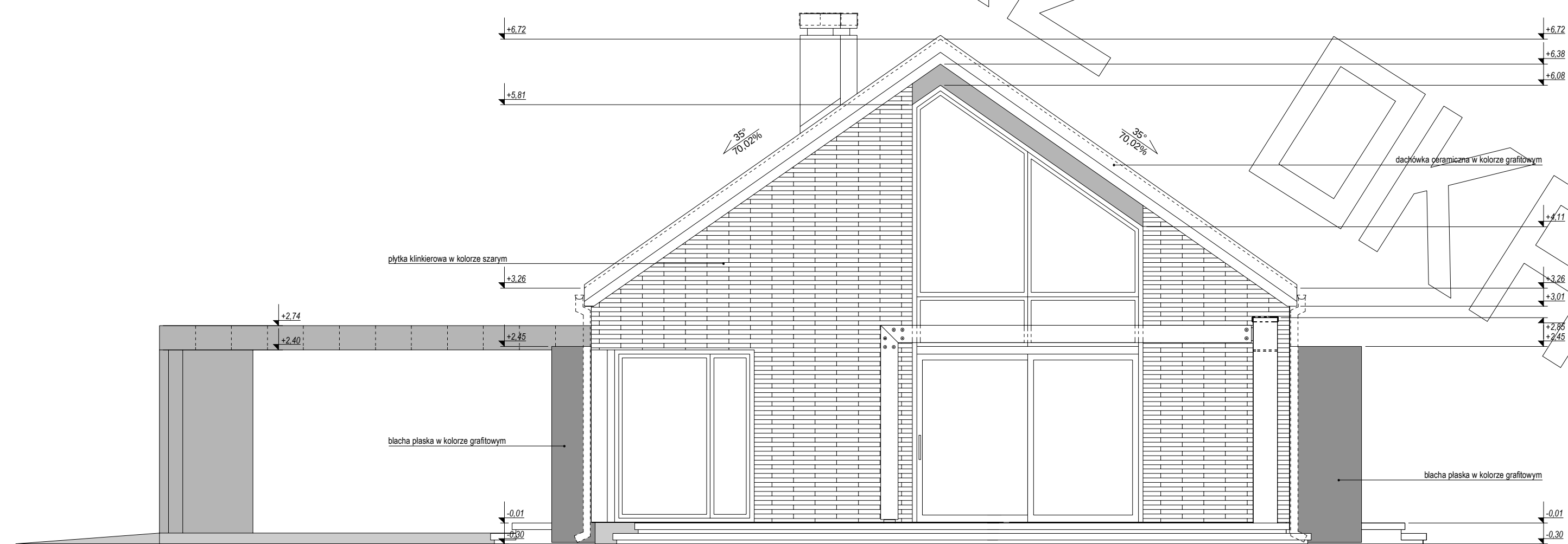
ELEWACJA BOCZNA:
