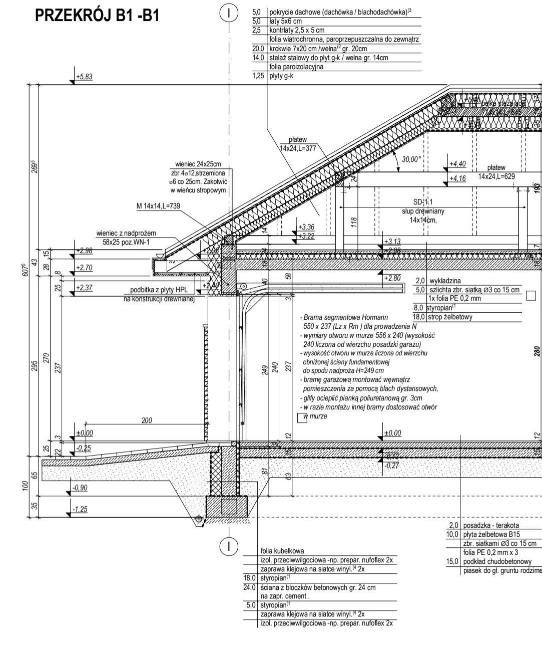
PRZEKRÓJ B1-B1
