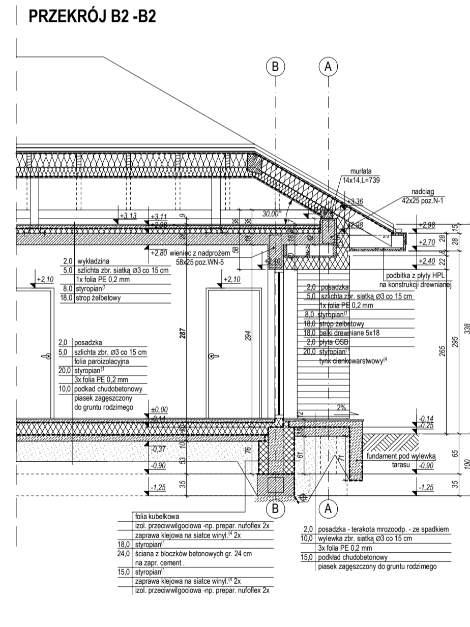
PRZEKRÓJ B2-B2
