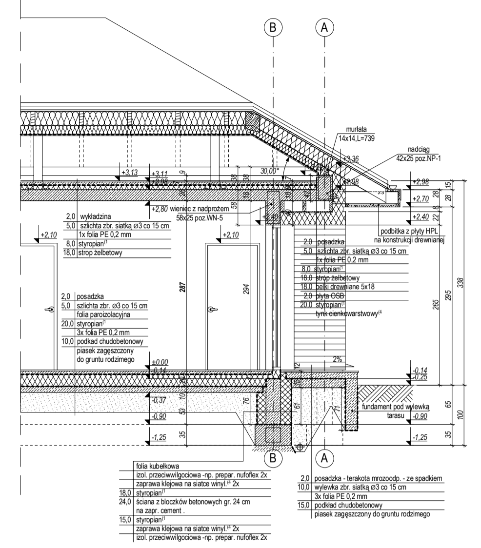
PRZEKRÓJ B2 - B2
