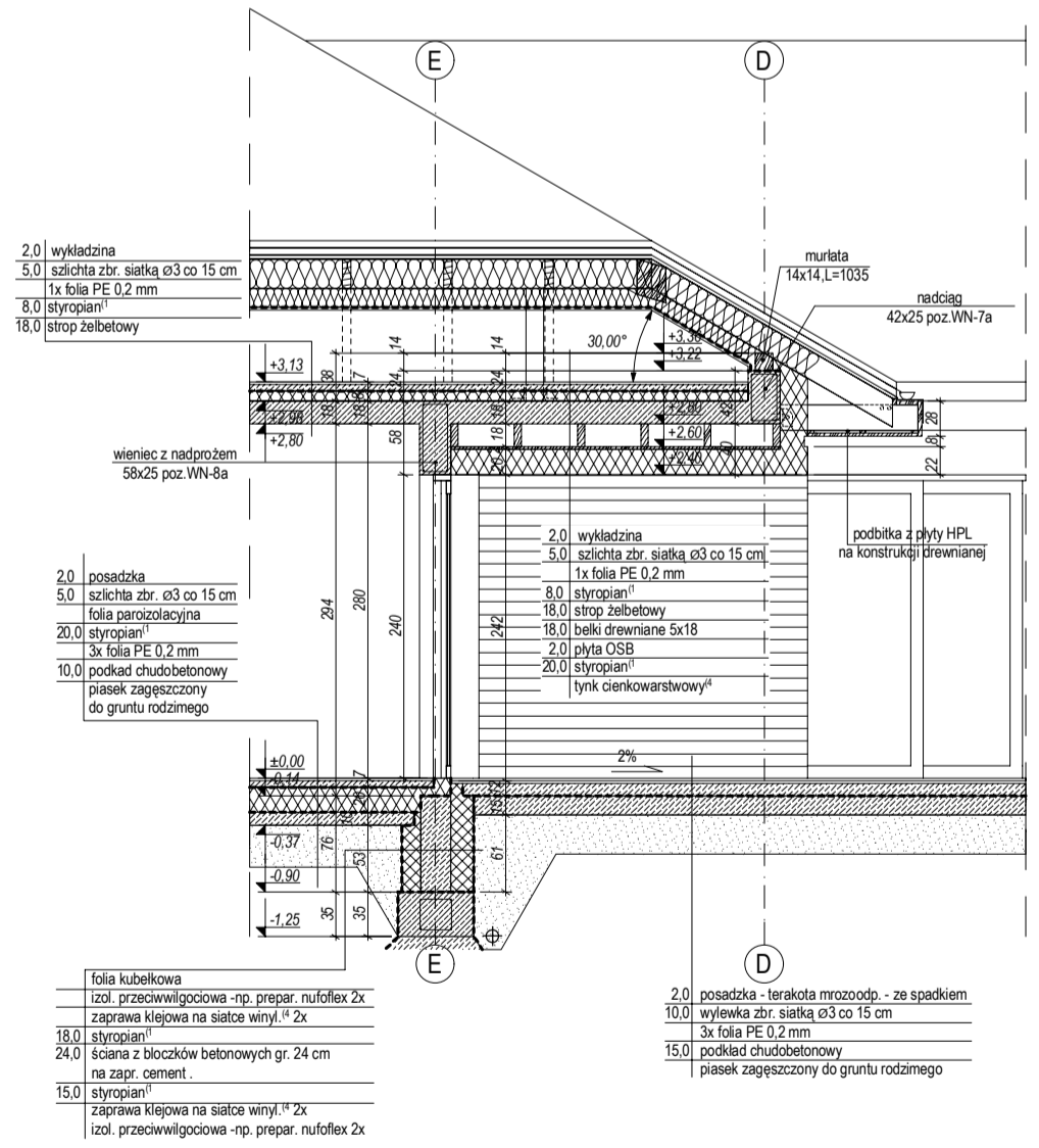
PRZEKRÓJ B3 - B3
