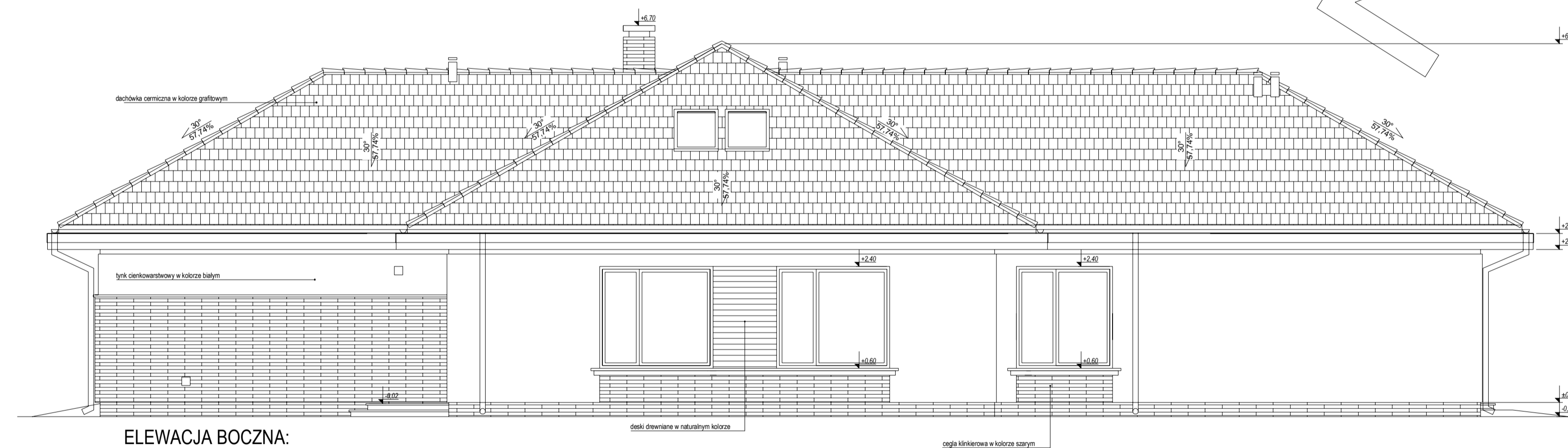
ELEWACJA BOCZNA:
