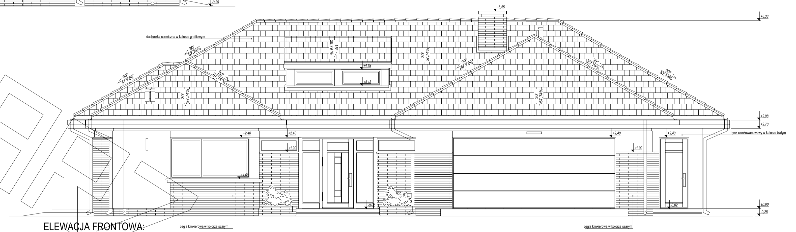
ELEWACJA FRONTOWA:
