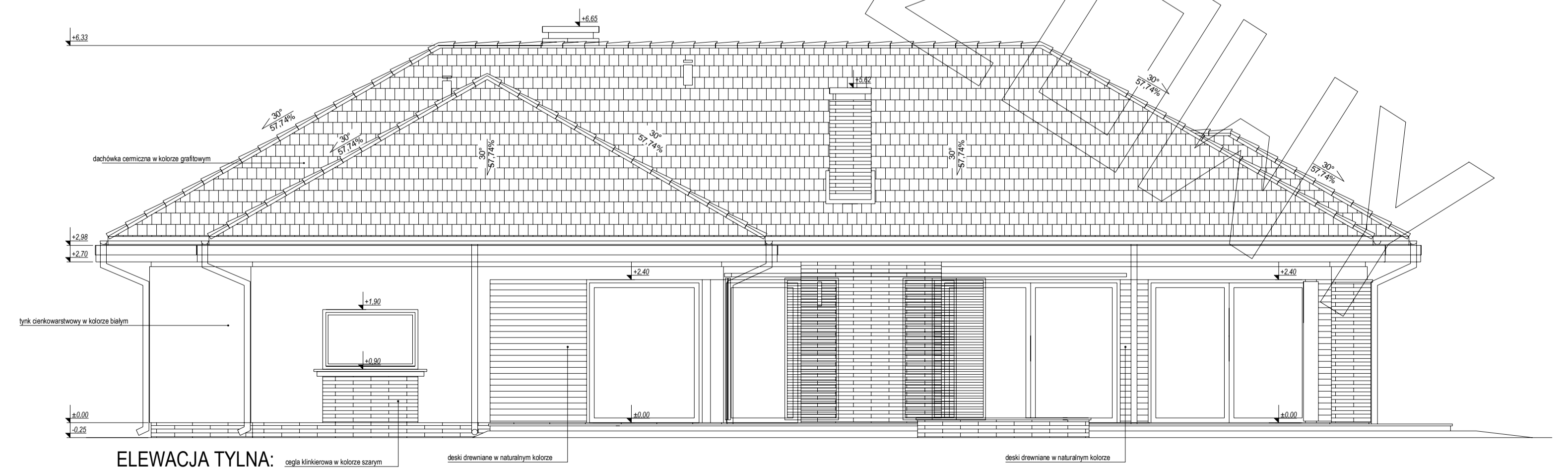
ELEWACJA TYLNA:
