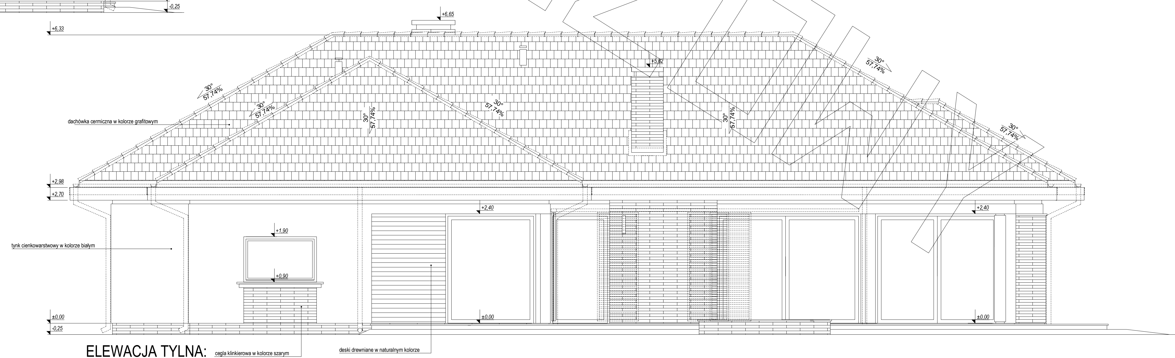
ELEWACJA TYLNA:
