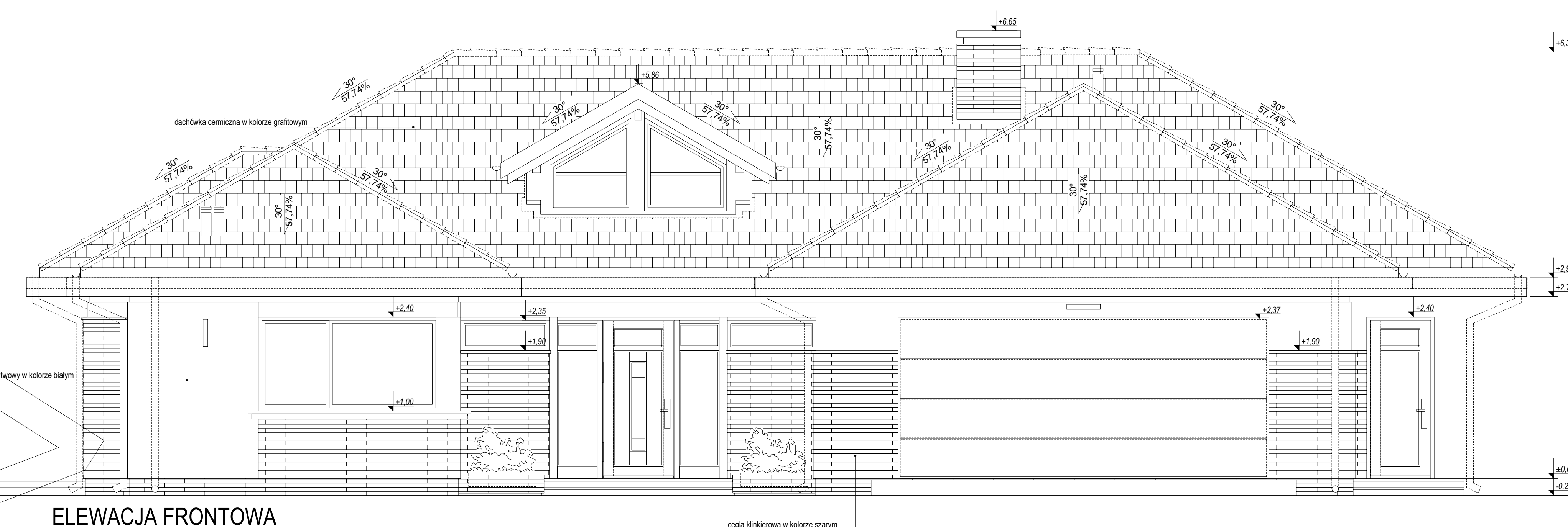
ELEWACJA FRONTOWA
