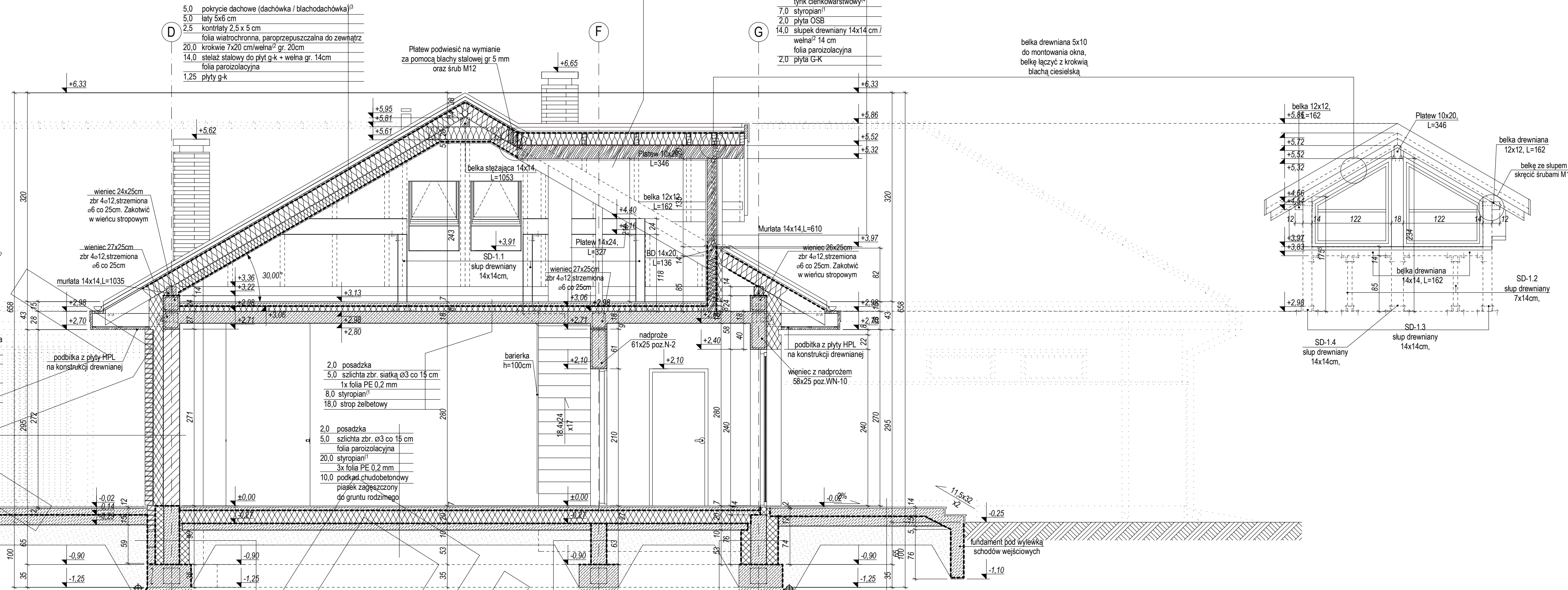
PRZEKRÓJ B - B
