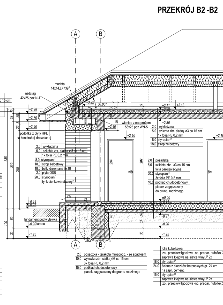
PRZEKRÓJ B2-B2
