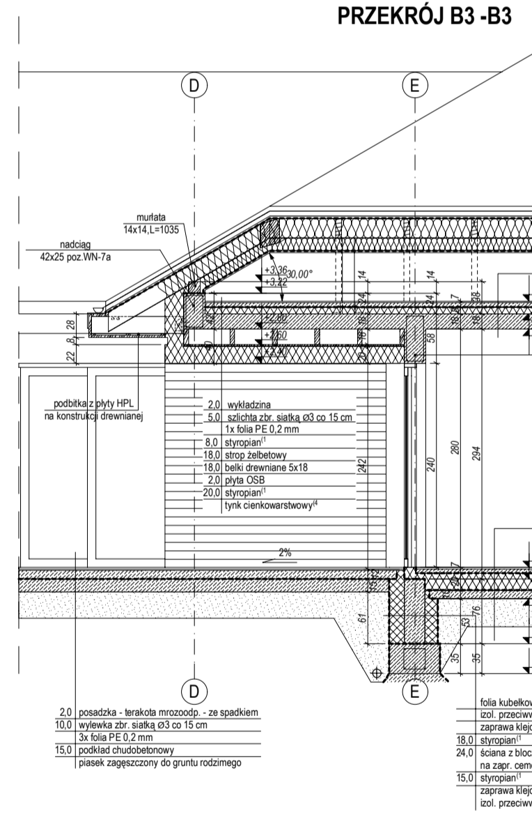
PRZEKRÓJ B3-B3
