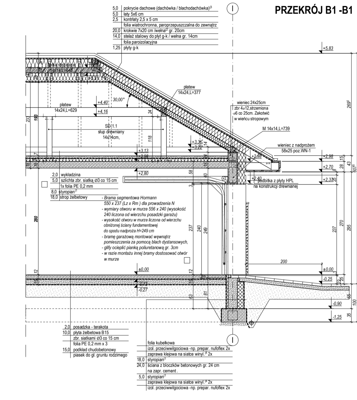
PRZEKRÓJ B1-B1
