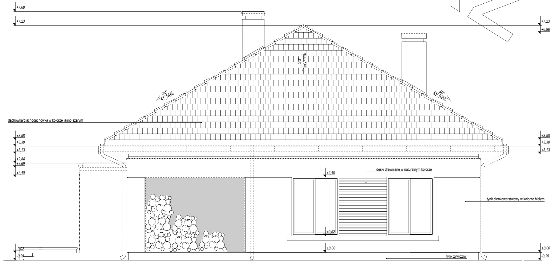
ELEWACJA TYLNA:
