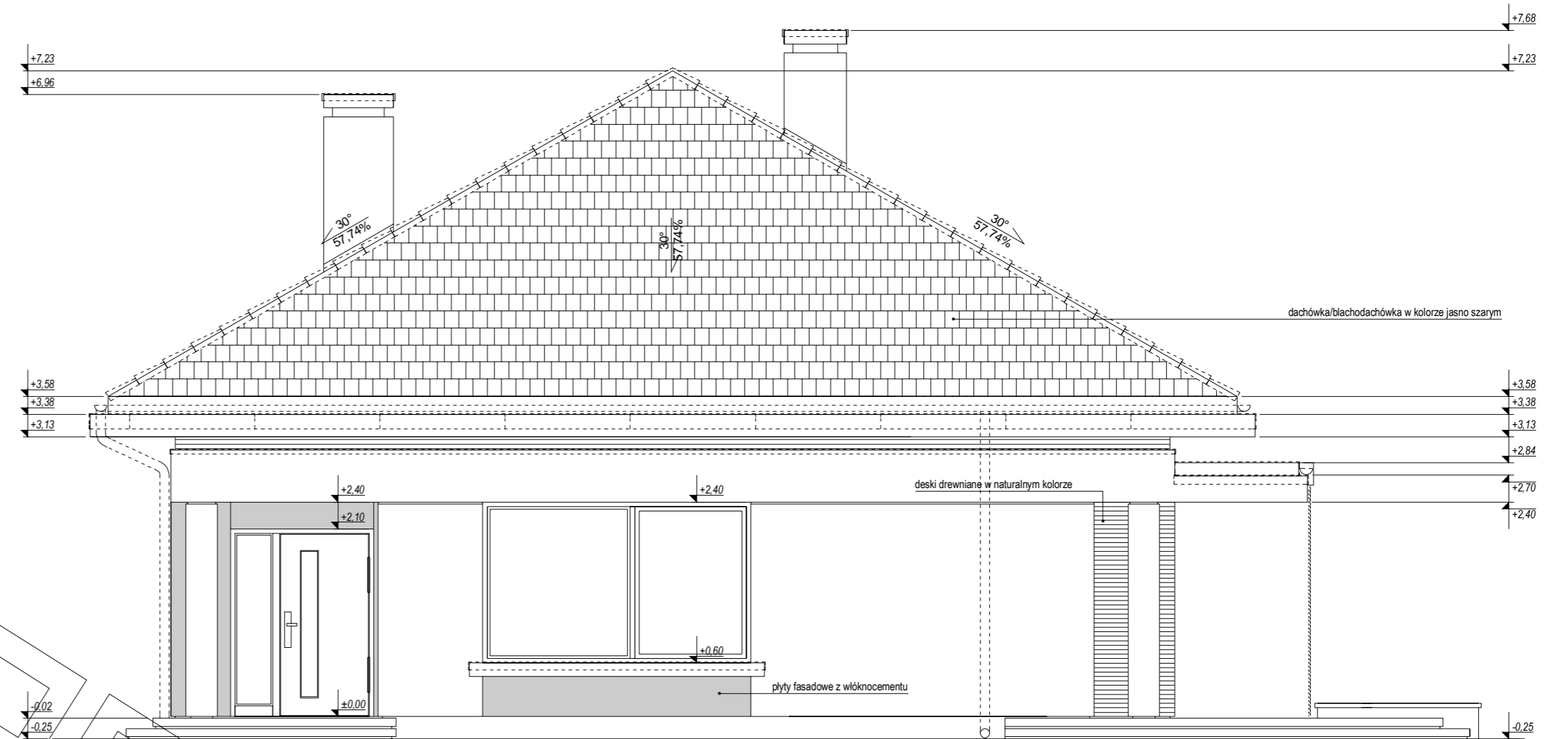
ELEWACJA FRONTOWA:
