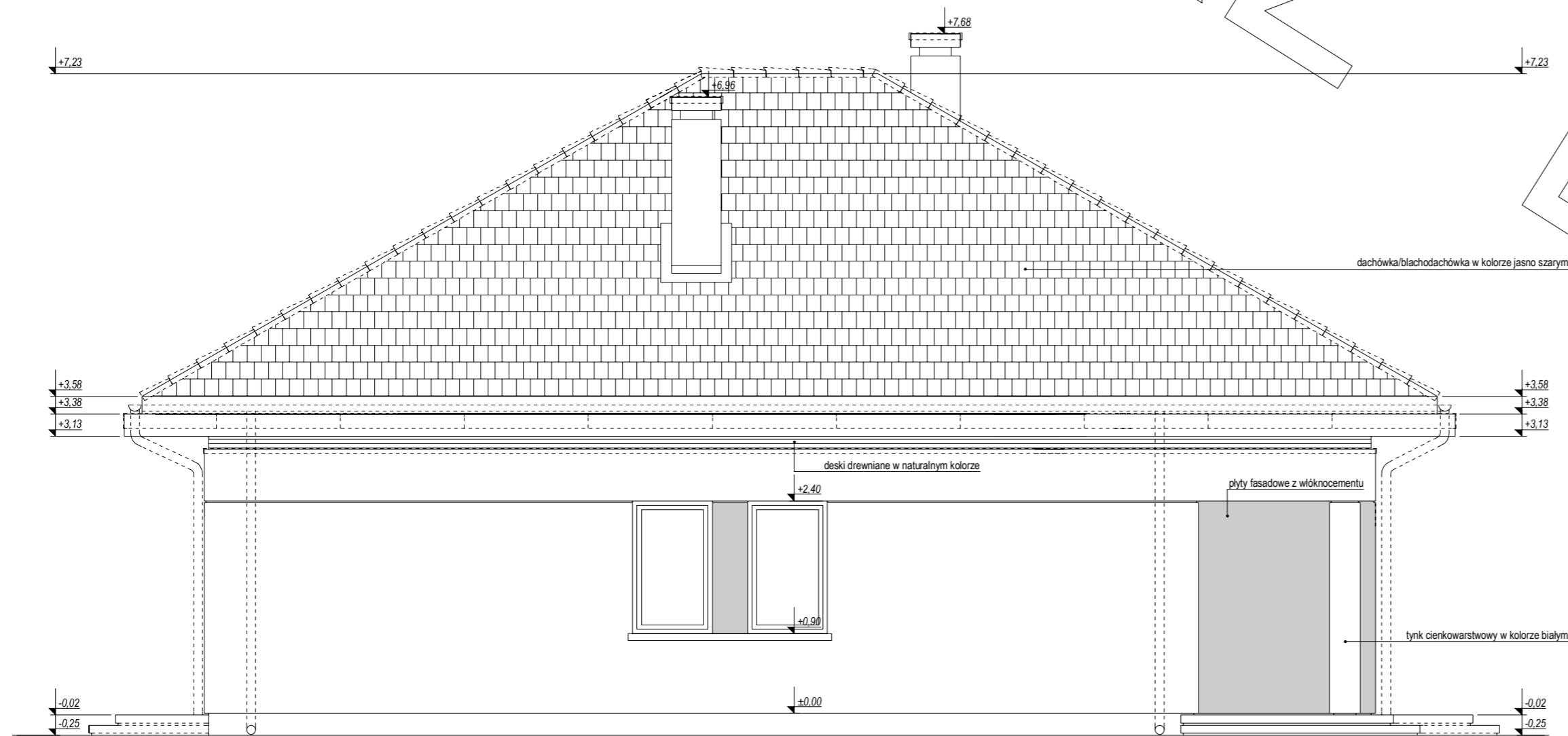
ELEWACJA BOCZNA:
