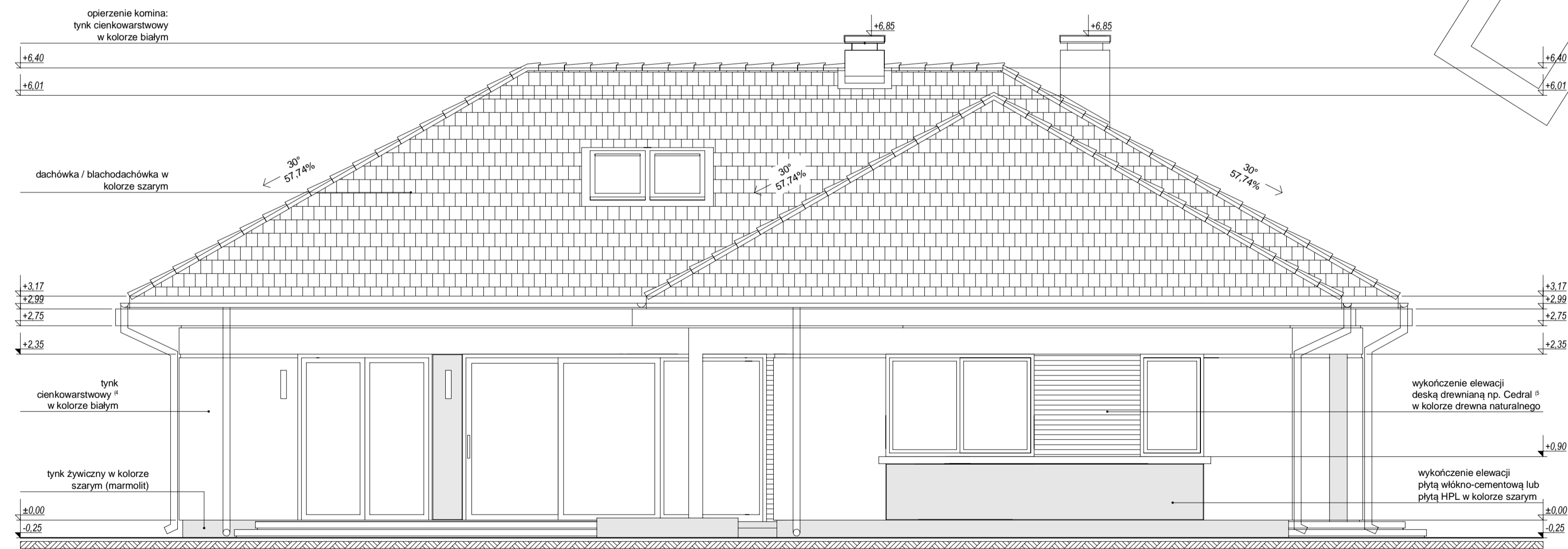
elewacja tylna :
