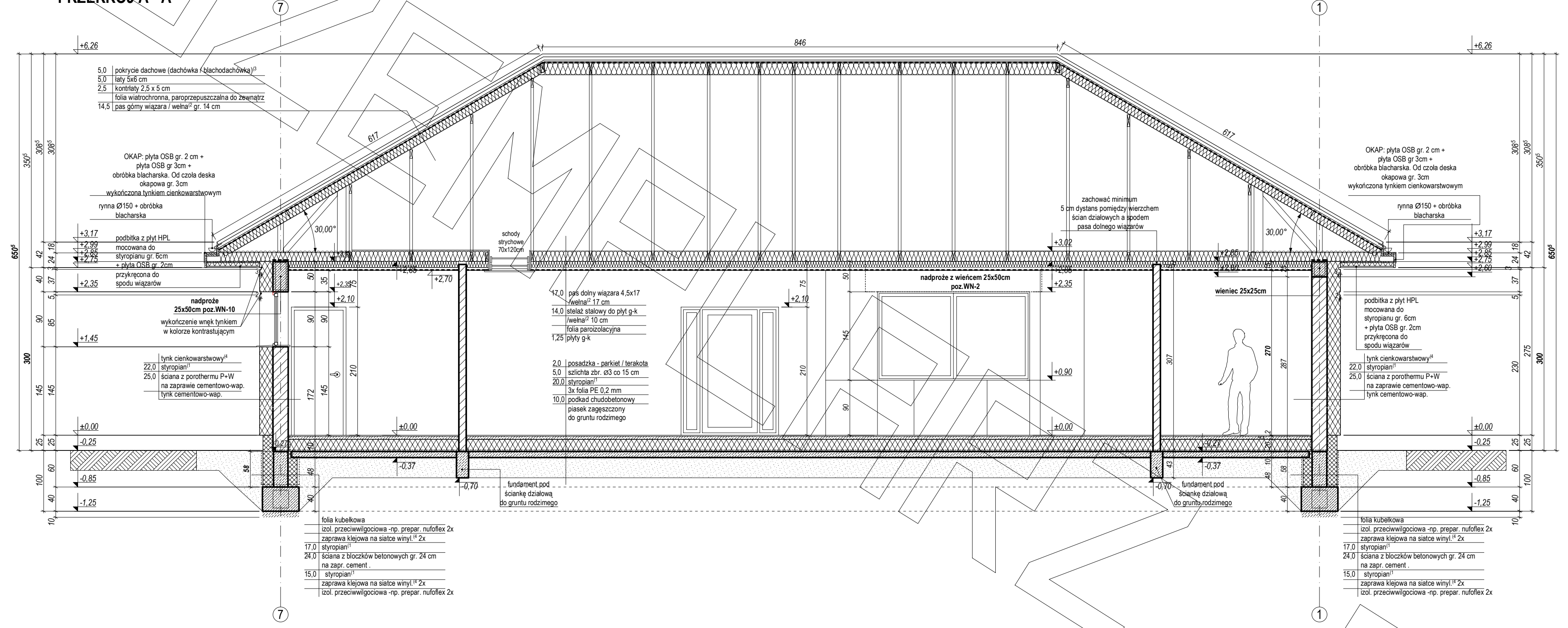
PRZEKRÓJ A - A
