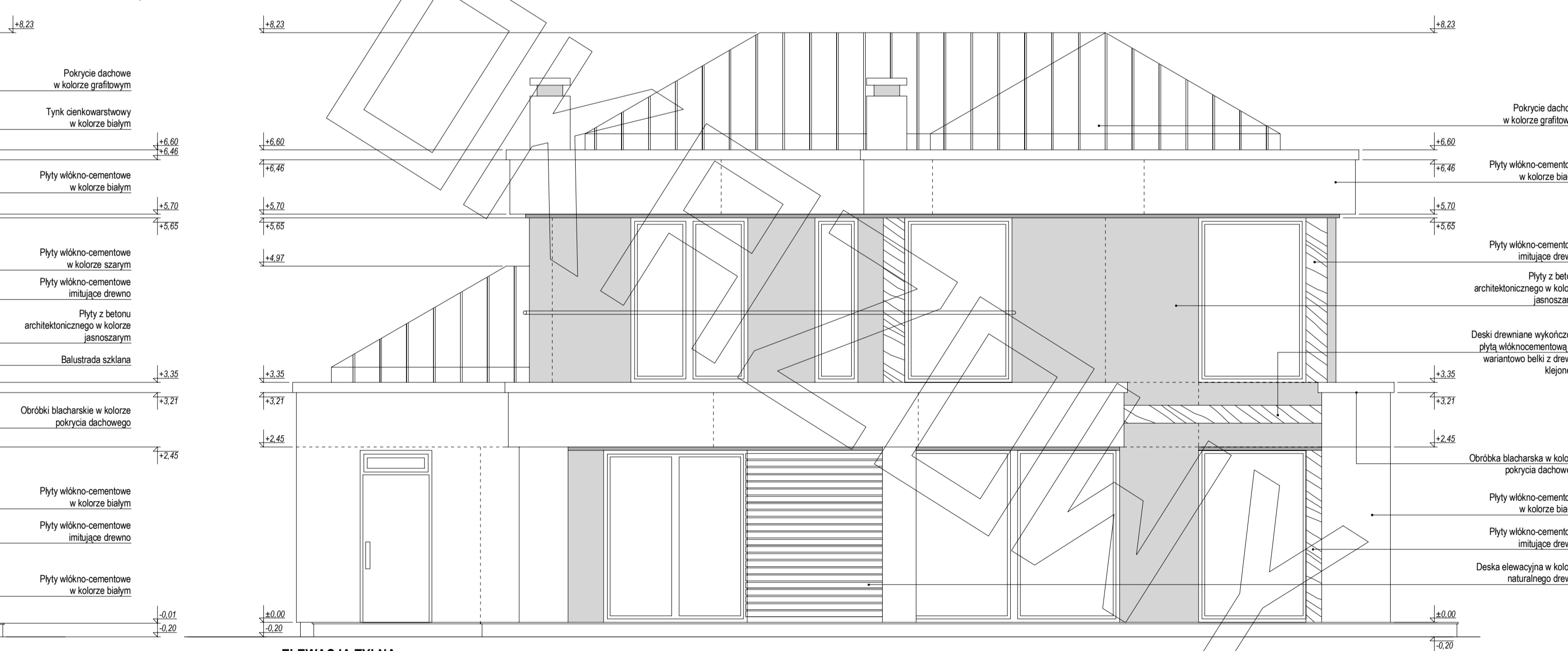
ELEWACJA TYLNA
