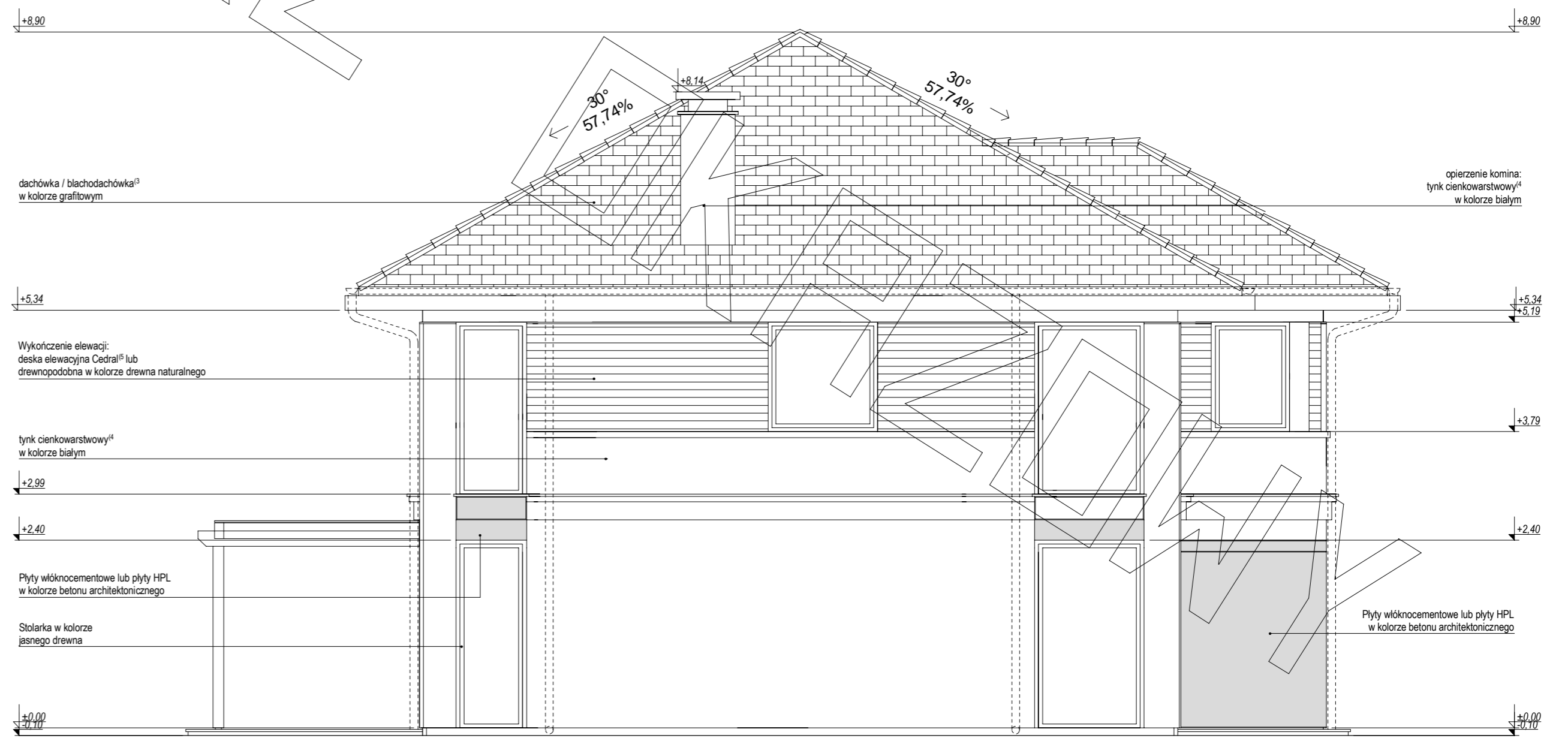
ELEWACJA BOCZNA
