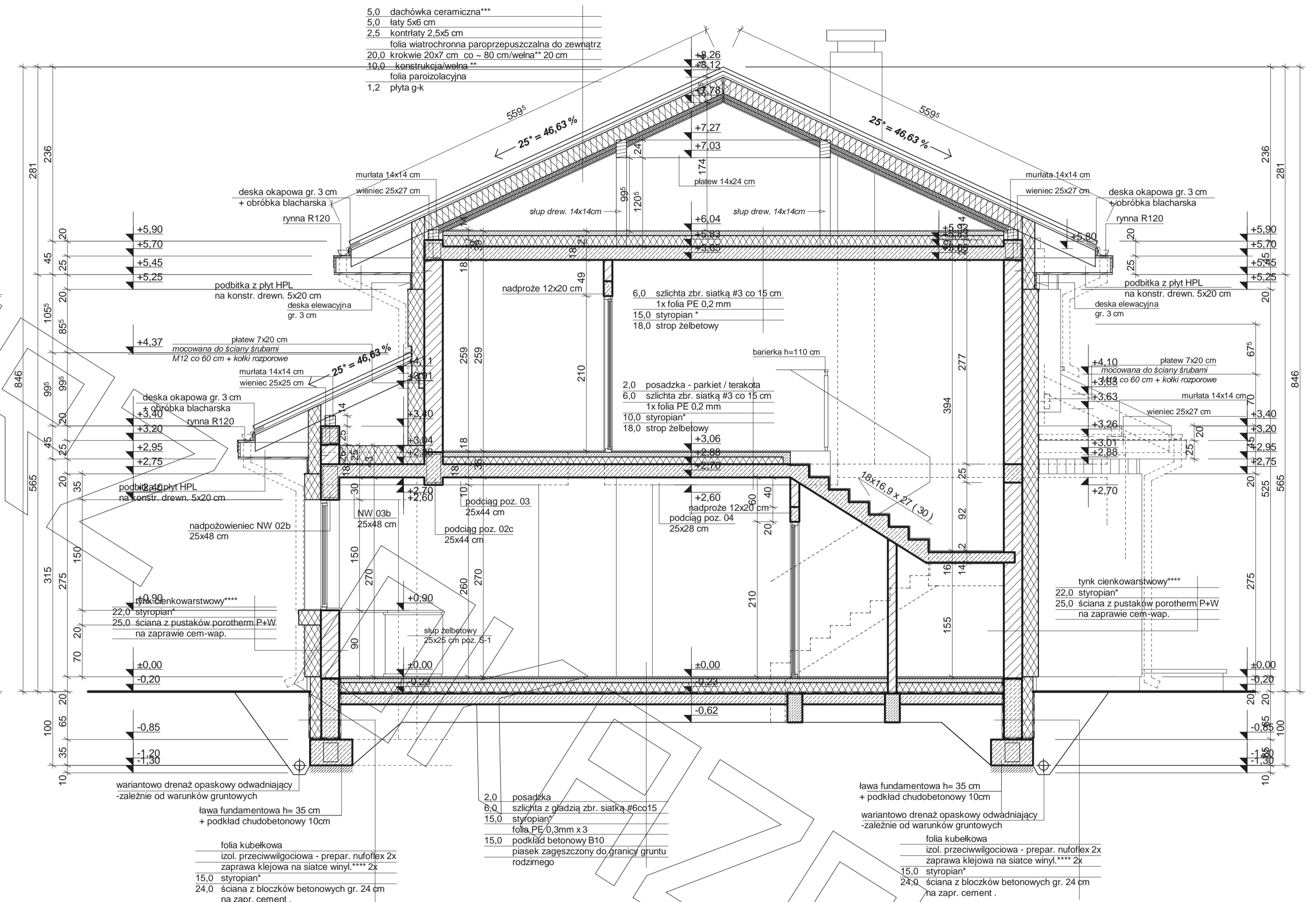
PRZEKRÓJ B-B
