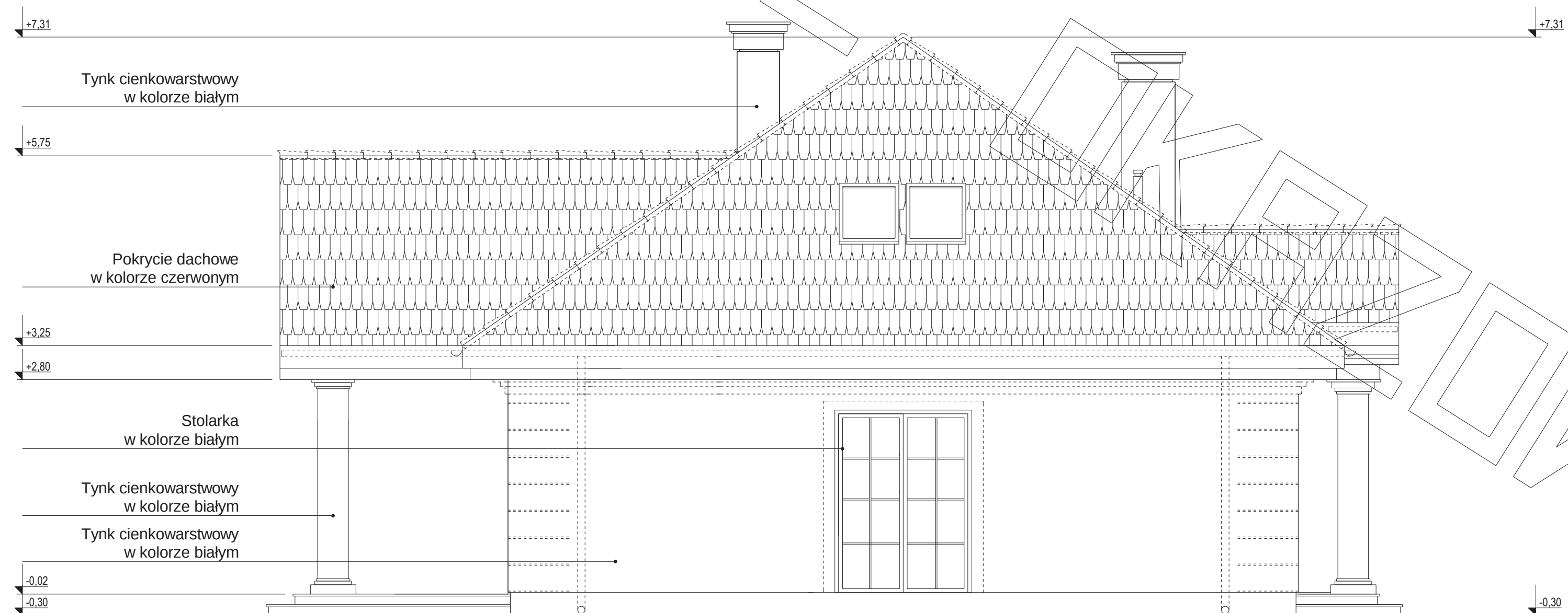
ELEWACJA BOCZNA
