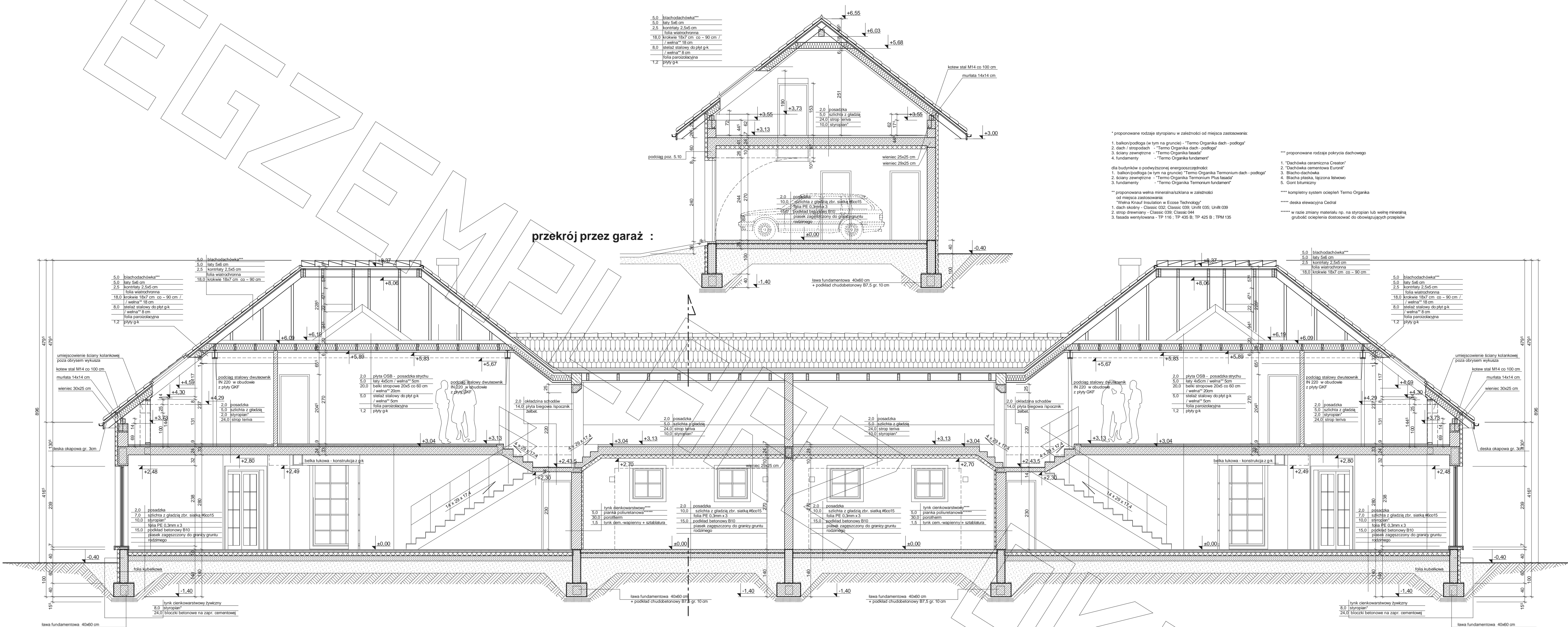
przekrój podłużny :
