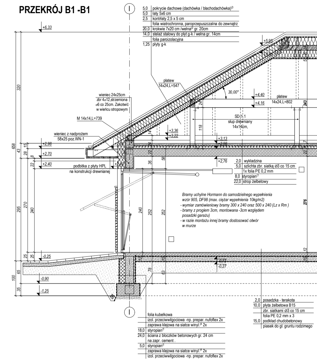
PRZEKRÓJ B1-B1
