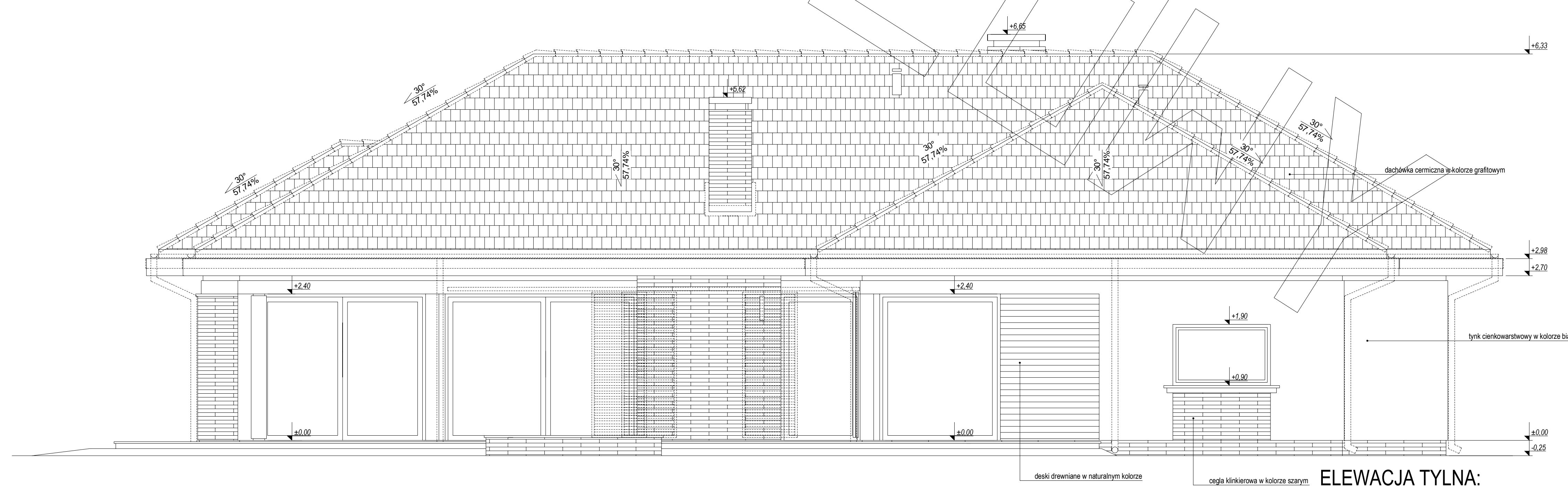
ELEWACJA TYLNA:
