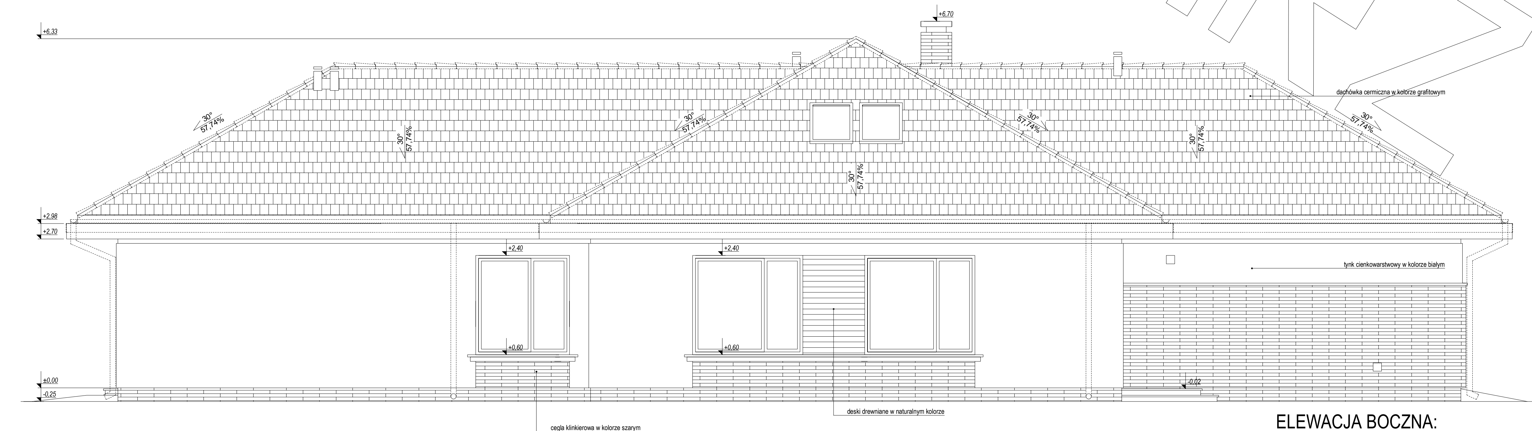
ELEWACJA BOCZNA:
