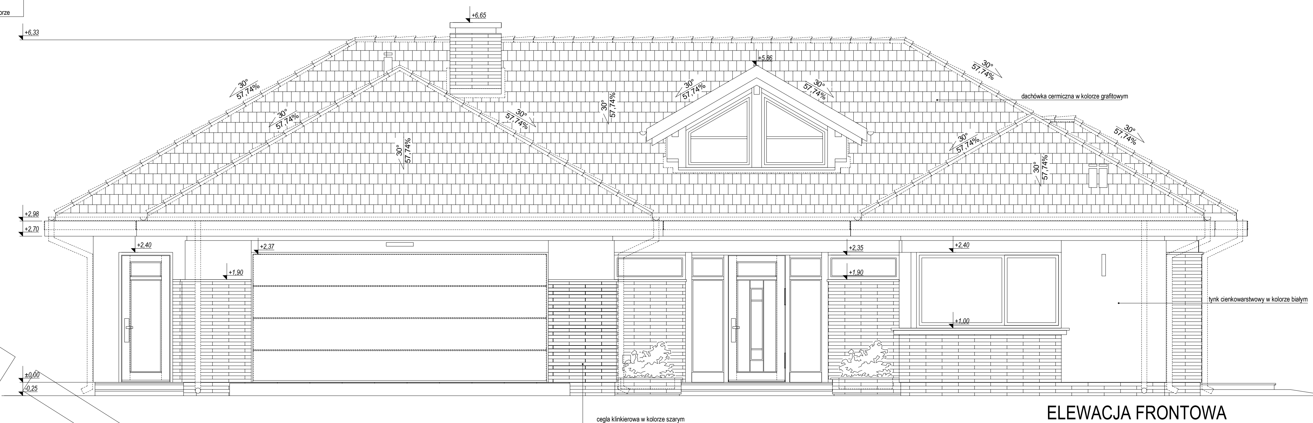
ELEWACJA FRONTOWA
