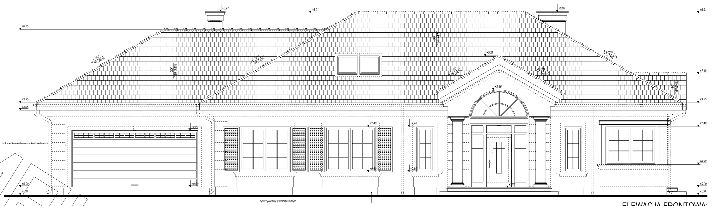
ELEWACJA FRONTOWA:
