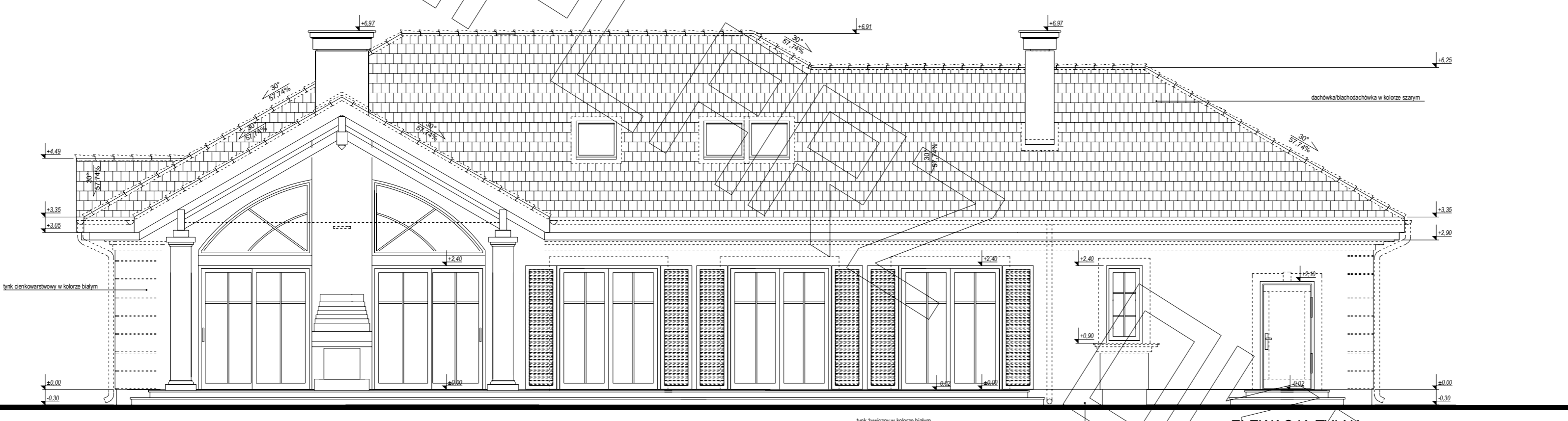
ELEWACJA TYLNA:
