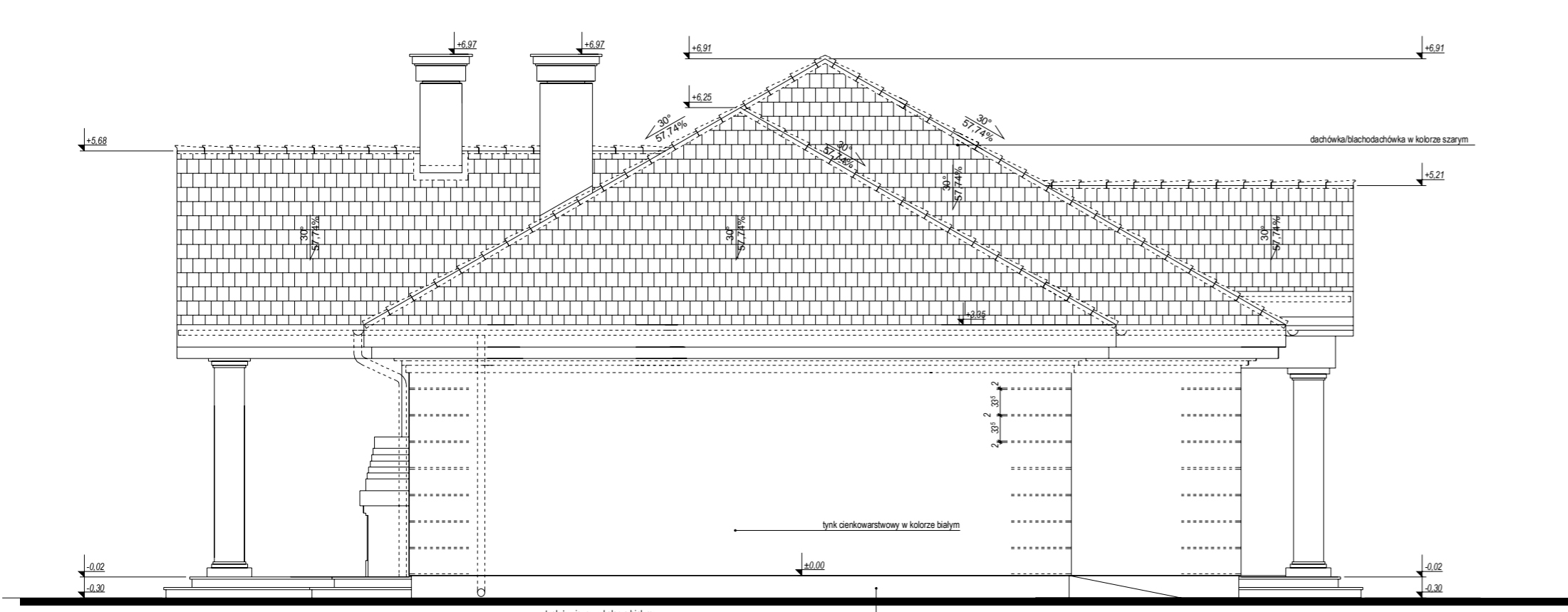
ELEWACJA BOCZNA:
