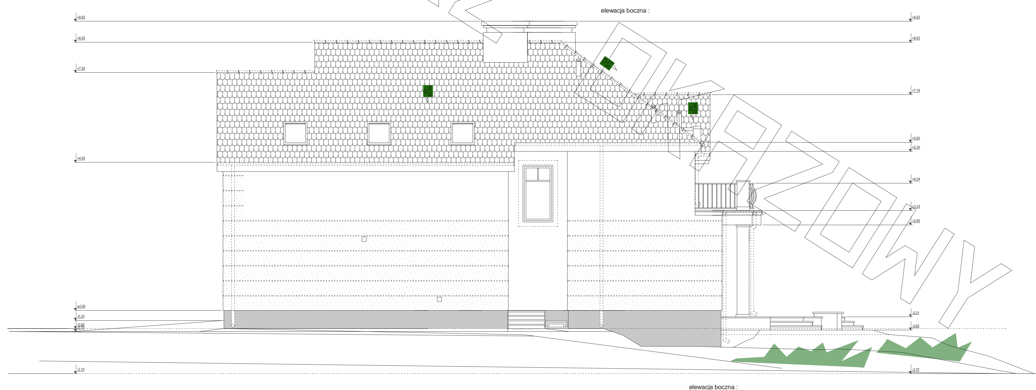
elewacja boczna :
