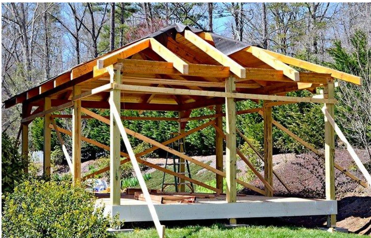
Budowa altany konstrukcja
