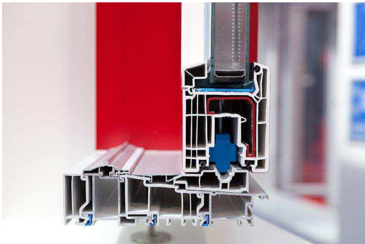
Okna plastikowe – przekrój
